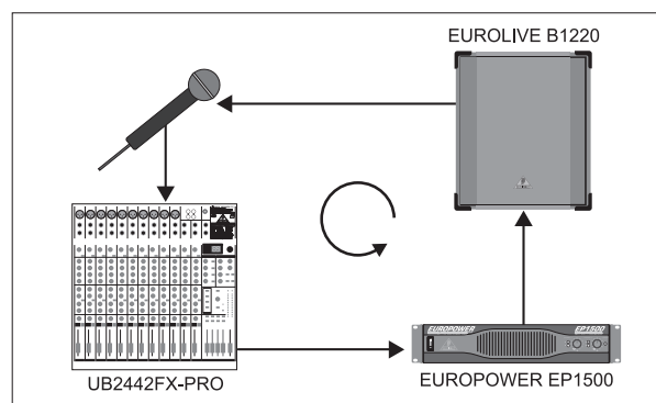
Εικ. 2.1: Δημιουργία ενός βρόχου ανάδρασης
