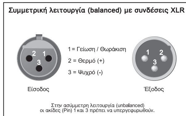
Εικ. 8.2: Βύσμα XLR
