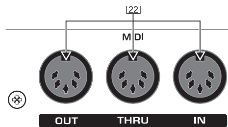
Εικ. 3.5: Υποδοχές σύνδεσης MIDI του FBQ2496
