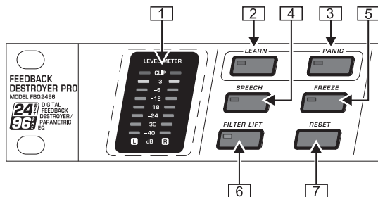
Εικ. 3.1: Στοιχεία χειρισμού στην αριστερή πλευρά του FBQ2496
