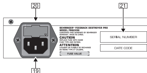
Εικ.3.4: Σύνδεση δικτύου, διακόπτης ασφαλείας και σειριακός αριθμός
