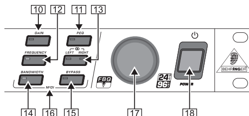
Εικ. 3.3: Στοιχεία χειρισμού στην δεξιά πλευρά του FBQ2496
