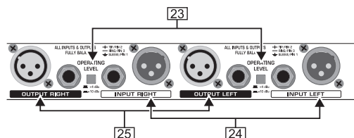
Εικ. 3.6: Συνδέσεις στην όπισθεν πλευρά του FBQ2496
