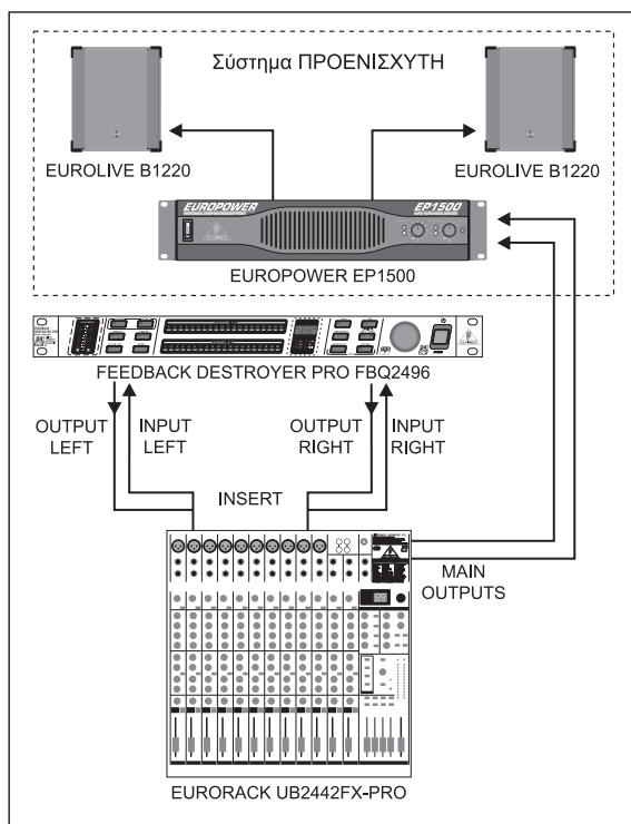
Εικ. 5.2: Ο FEEDBACK DESTROYER PRO στο Insert καναλιού και στο Insert υποομάδων
