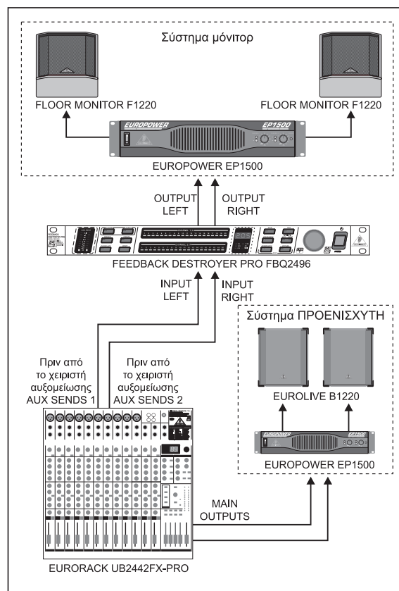
Εικ. 5.1: Χρήση του FBQ2496 στην οδό μόνιτορ
