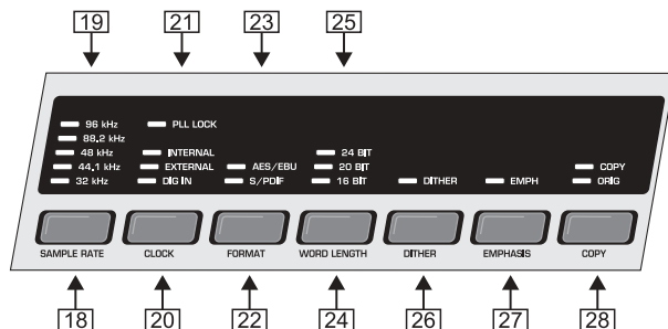
Εικ. 2.5: Το τμήμα εξόδου
