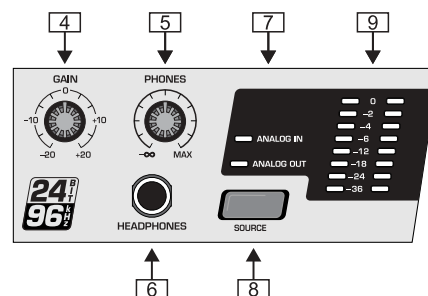
Εικ. 2.2: Στοιχεία χειρισμού του τμήματος εισόδου
