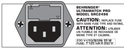
Εικ. 2.6: Πίσω πλευρά του ULTRAMATCH PRO
