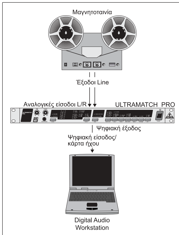
Εικ. 3.2: Παράδειγμα μετατροπής A/D παλαιότερων ηχογραφήσεων μαγνητοταινίας
