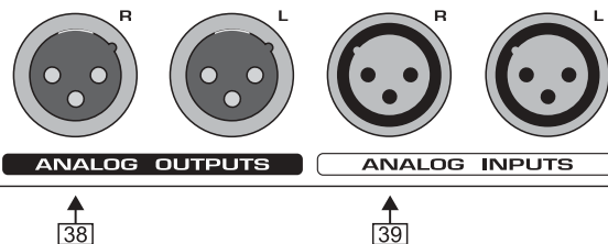
Εικ. 2.11: Αναλογικές εξόδοι / Αναλογικές εισόδοι
