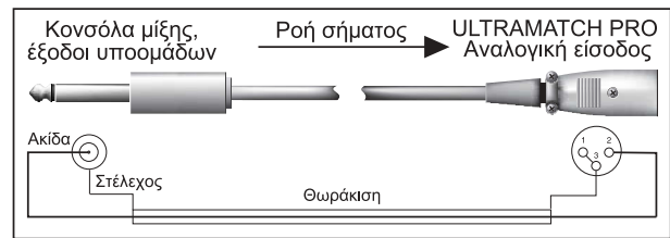
Εικ. 4.1: Ασύμμετρη αποστολή σήματος στον ULTRAMATCH PRO
