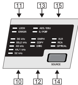
Εικ. 2.3: Στοιχεία χειρισμού του τμήματος εισόδου
