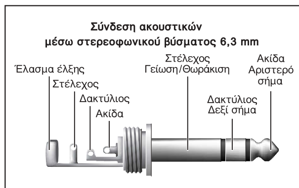
Εικ. 4.7: Σωστή αντιστοίχιση για τη μετάδοση σήματος στα ακουστικά
