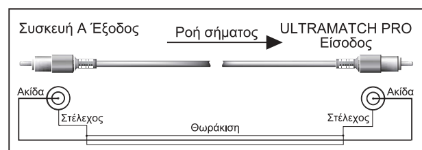
Εικ. 4.4: Ασύμμετρος τρόπος σύνδεσης του ULTRAMATCH PRO
