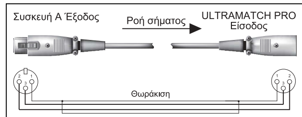
Εικ. 4.3: Συμμετρικός τρόπος σύνδεσης του ULTRAMATCH PRO
